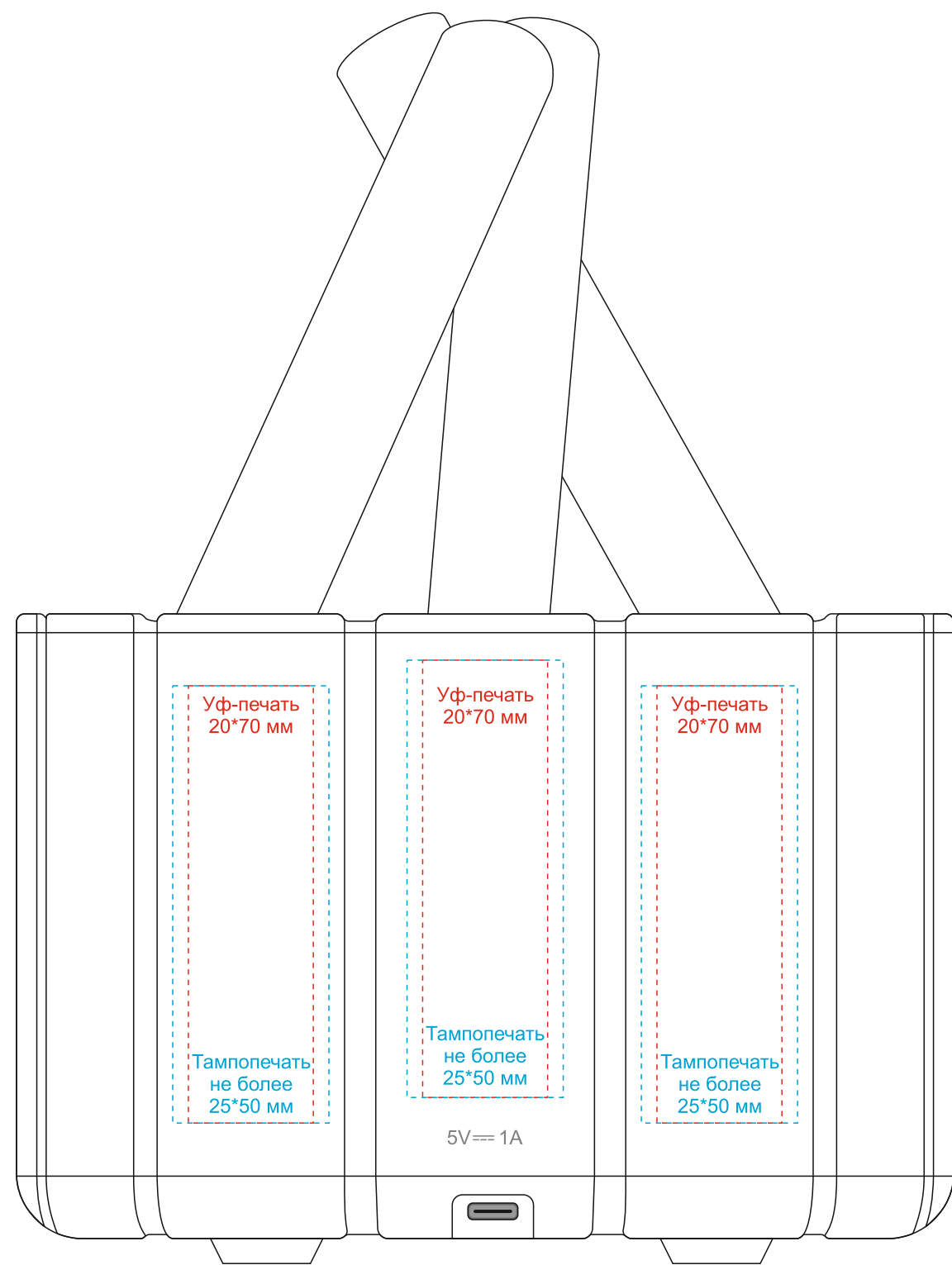
Вид сзади
