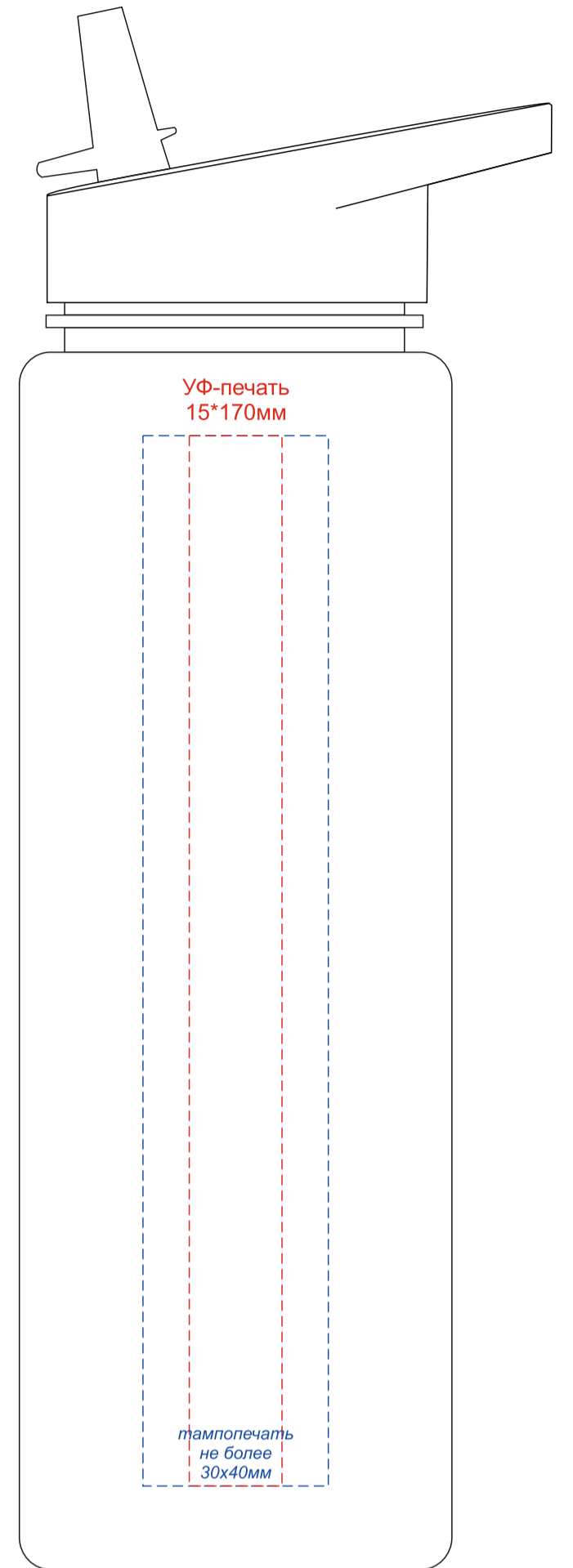
вид справа
