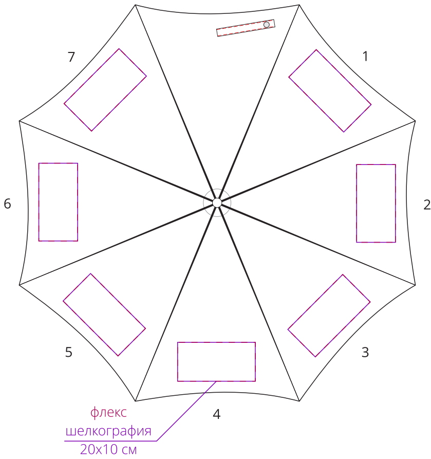
купол M1:10
