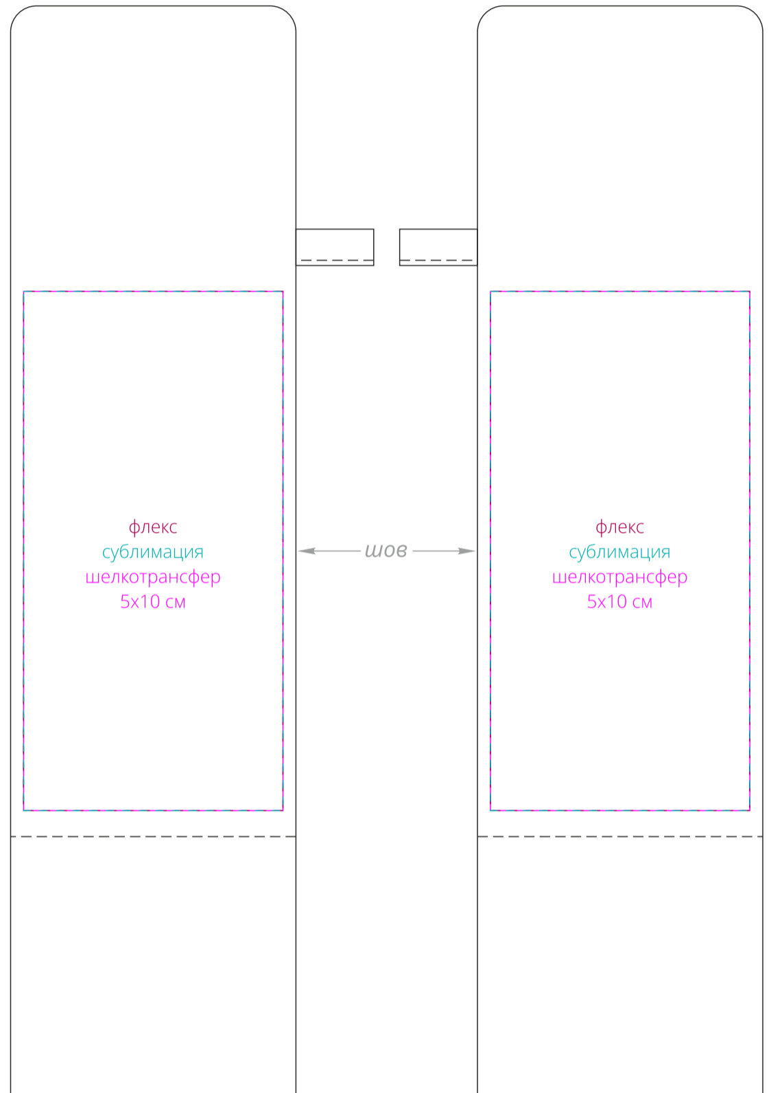
чехол M1:1
