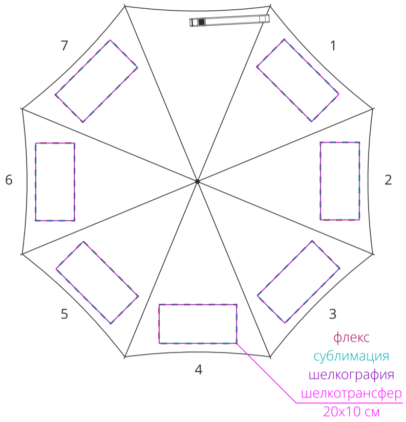
купол M1:10
