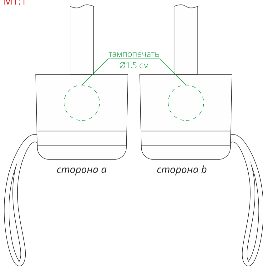
ручка M1:1
